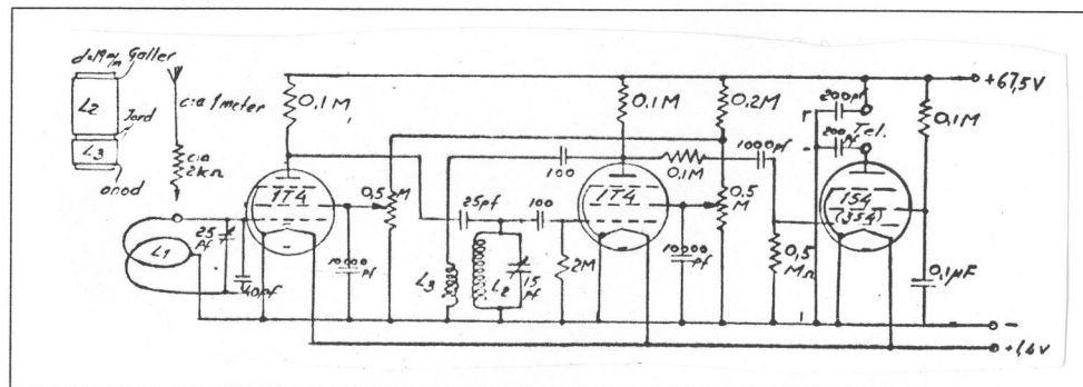
Rävmottagare med rör, QRZ, april 1949.
